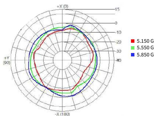
H-Plane
