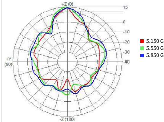
E-Plane
