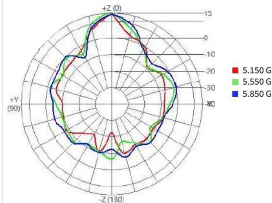
E-Plane
